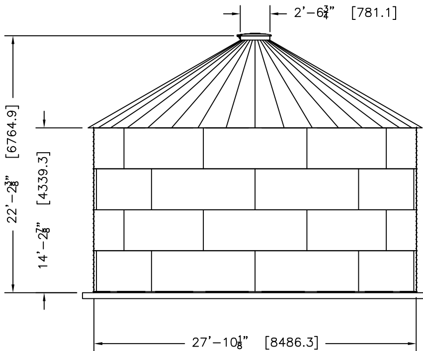
ELEVATION
